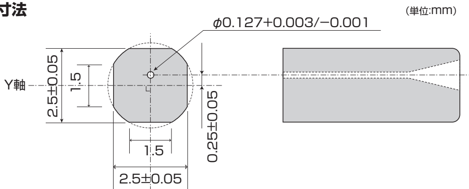
従来構造
